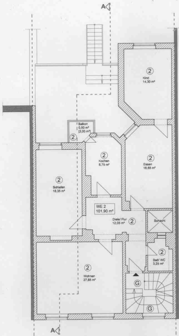
1. OBERGESCHOSS
