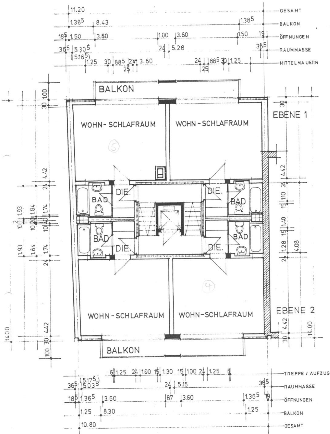
1. OBERGESCHOSS (EB. 1 + 2)
